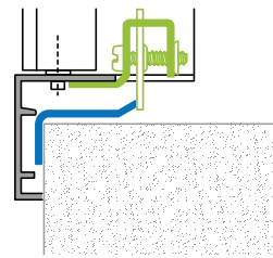
Fissaggio con morsetti
