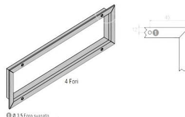
① Ø 3,5 Foro svassetto
