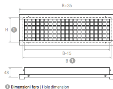
① Dimensioni foro | Hole dimension
