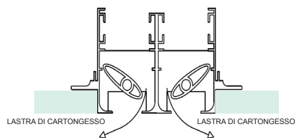
LANCIO ORIZZONTALE DIREZIONI OPPOSITE
