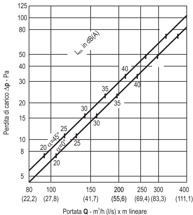
DLSC 2 feritoie Dp e L_{WA}
