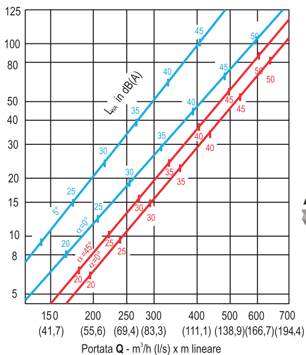
DLSC 4 feritoie (■) e 3 feritoie (■) Dp e L_{WA}
