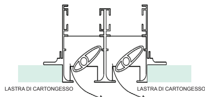
LANCIO ORIZZONTALE STESSA DIREZIONE
