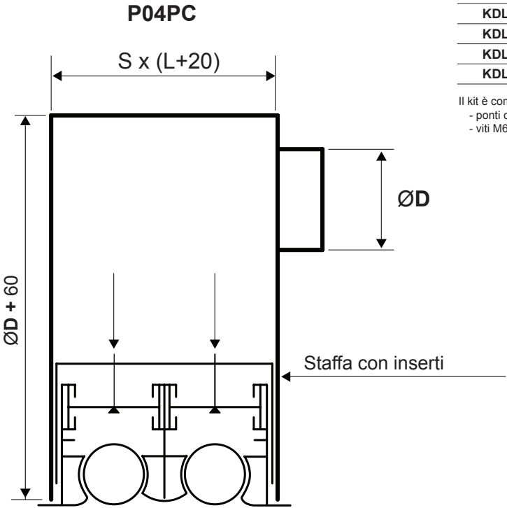
Fissaggio al plenum con staffe e viti
