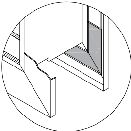
PARTICOLARE DELL'INSERIMENTO TELAIO CONTROTELAIO
