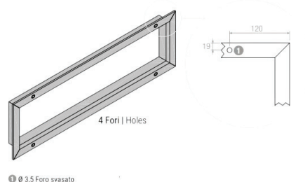
① Ø 3,5 Foro svasato
